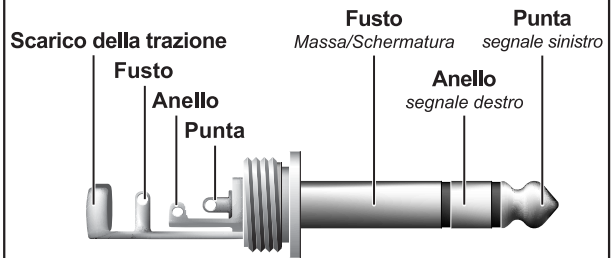
Fig. 4.4: Presa jack stereo per cuffia
