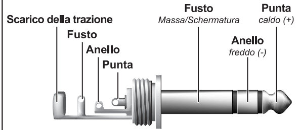
Fig. 4.3: Presa jack stereo 6,3 mm
