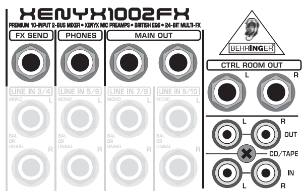
Fig.2.3: I collegamenti della sezione main
