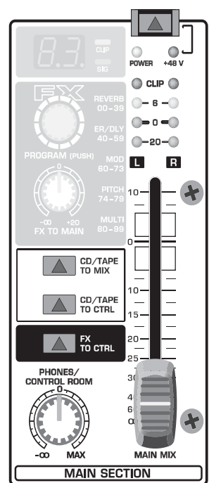
Fig. 2.4: Gli elementi di comando della sezione principale
