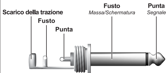
Fig. 4.2: Presa jack mono 6,3 mm
