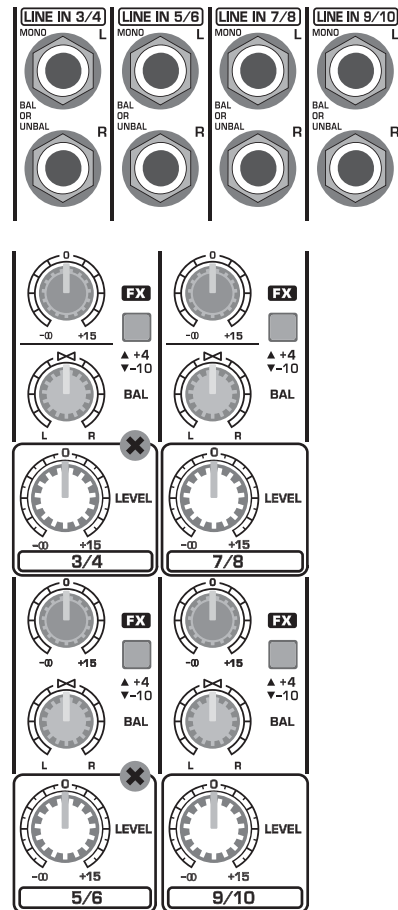
Fig. 2.2: I collegamenti ed i regolatori dei canali stereo
